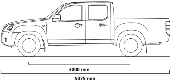
Четырехдверная кабина
